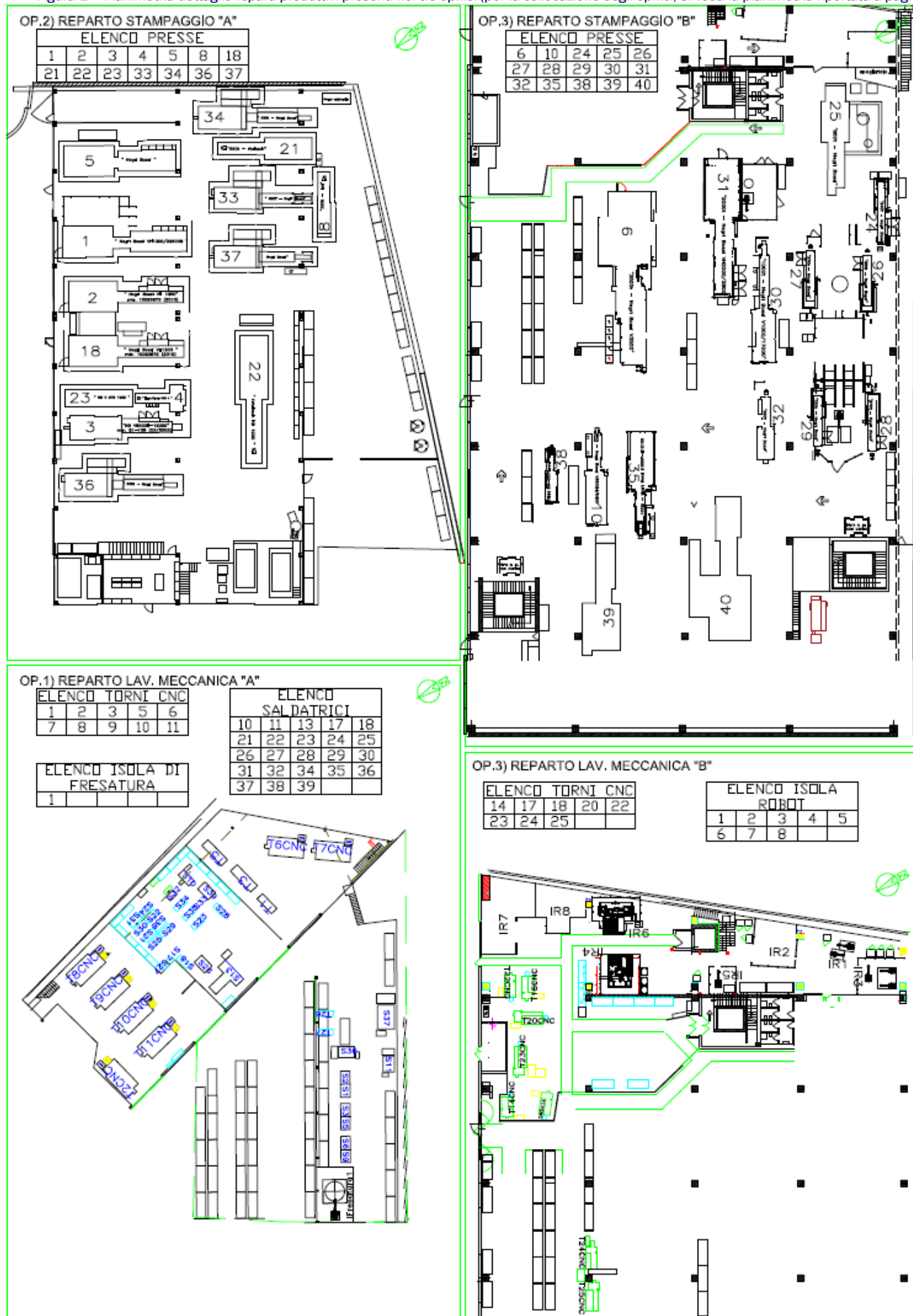
Figura 1 – Planimetria dettaglio reparti produttivi presenti nei tre opifici (per la collocazione degli opifici, si veda la planimetria riportata a pag.8)
