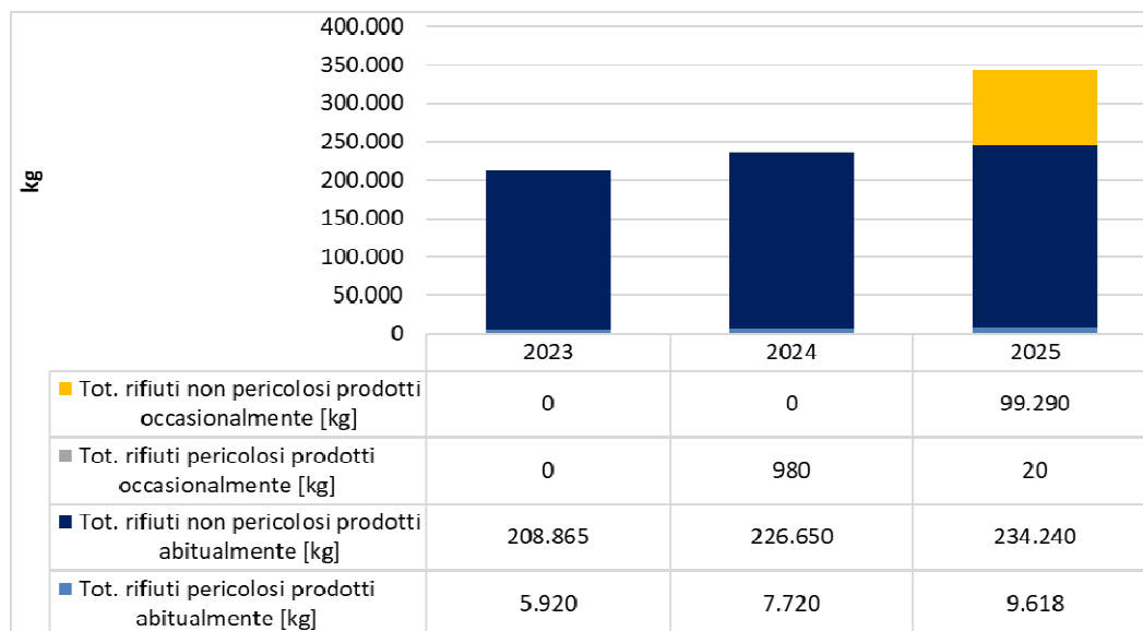
Figura 2 – Quantità rifiuti pericolosi e non pericolosi prodotti dal 2023 al 2025
