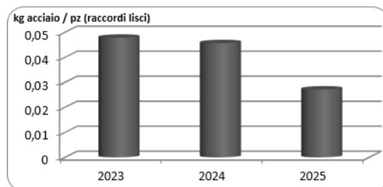
Figura 7 – Acciaio consumato / pz prodotti (raccordi lisci) (dal 2023 al 2025)
