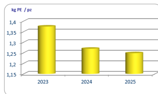
Figura 6 – Materia prima consumata / pz prodotti (dal 2023 al 2025)
