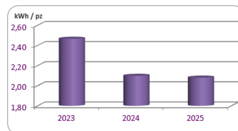
Figura 5 – Energia consumata / pz prodotti (dal 2023 al 2025)
