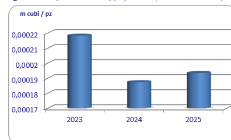
Figura 1 – Acqua consumata/pz prodotti (dal 2023 al 2025)
