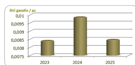
Figura 2 – Gasolio consumato / pz prodotti (dal 2023 al 2025)
